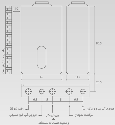
وضعیته اتصالات دستگاه
