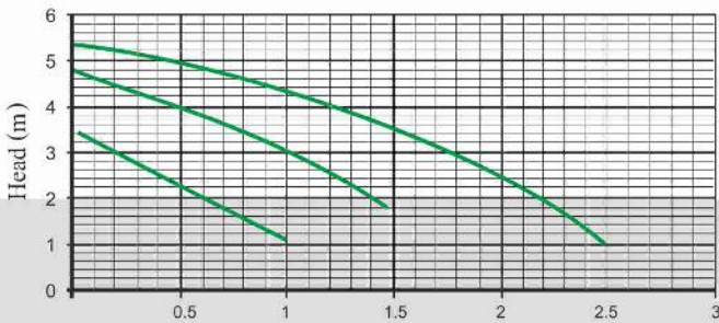
مشخصات هیدرولیکی MSL 12/5-3
