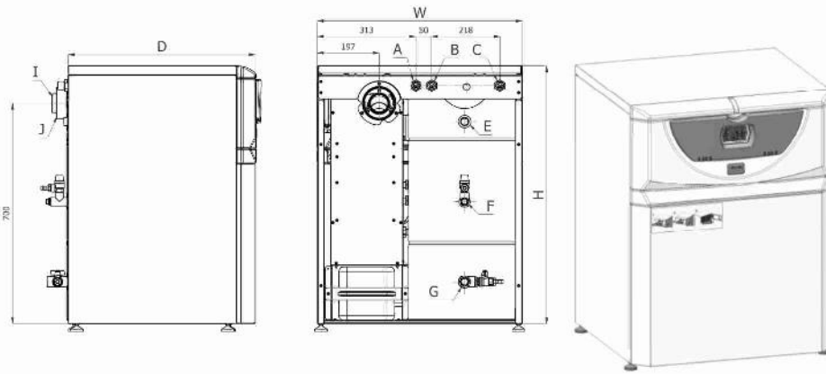
مشخصات هیدرولیکی MSL 12/5-3
