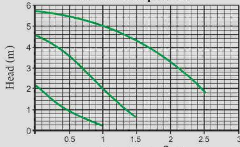
منحنی عملکرد پمپ ثانویه مدار شوقاژ
