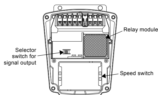
Fig. 11 Relay module
