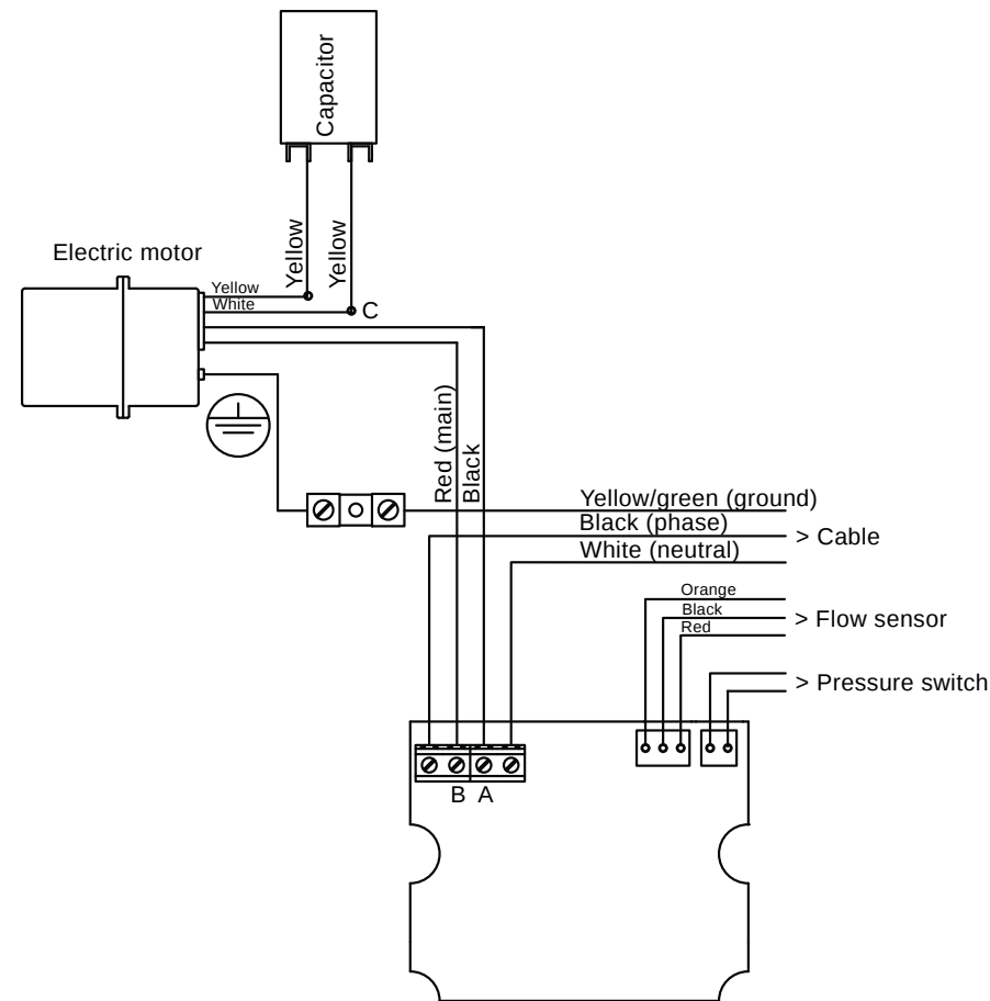
Fig. 12 Wiring diagram - 115 V
